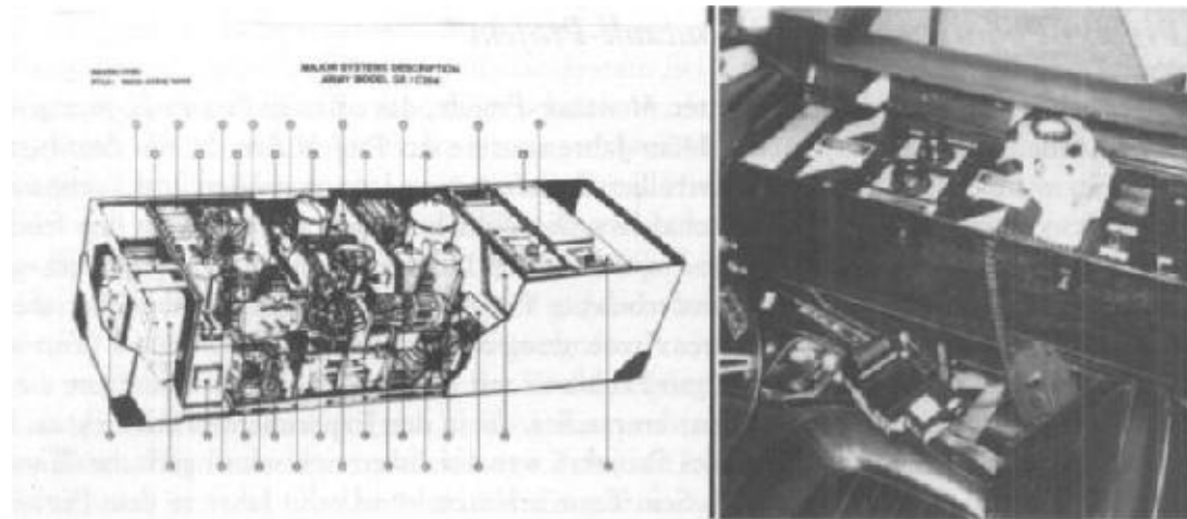
Abb. 276 und 277: Skizze der Zeitmaschine und das Gerät in der 1967er Corvette
